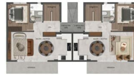
ZEMİN KAT PLANI
