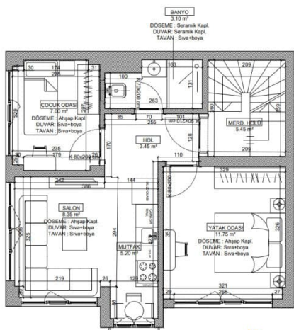
1. KAT PLAN
